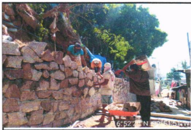
MURO DE PIEDRA BRAZA
