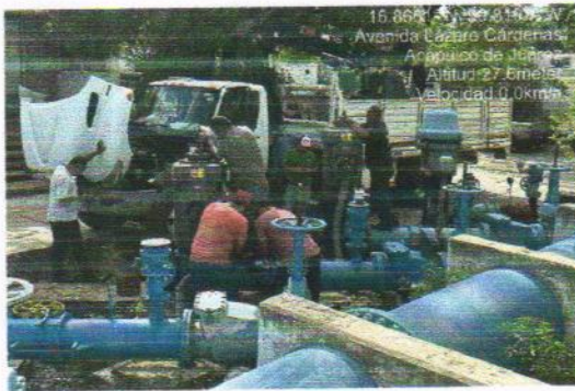
OBRA TERMINADA MOTOR 200 HP
