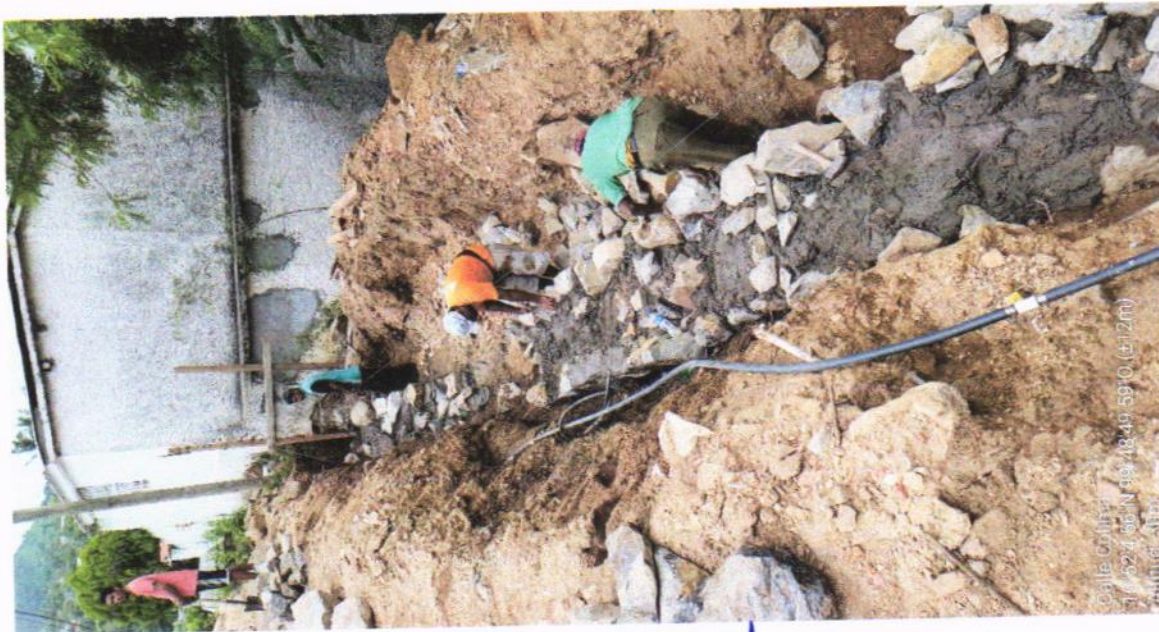
18-0294 MURO DE PIEDRA BRAZA DE LA REGION, ASENTADA CON MORTERO CEMENTO-ARENA 1:3, ACABADO COMUN, INCLUYE: ACARREO DE MATERIALES EN 1ra. ESTACION DE 20.00 MTS.
