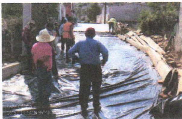
SUMINISTRO Y COLOCACIÓN DE MEMBRANA DE POLIETILENO
