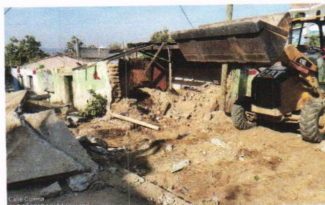
DEMOLICIÓN DE PAVIMENTO DE CONCRETO SIMPLE
