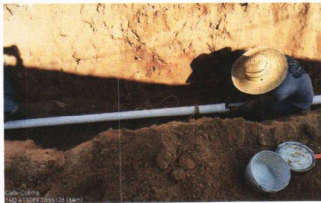
SUMINISTRO Y TENDIDO DE TUBERÍA DE 3" DE PVC CED. RD-26
