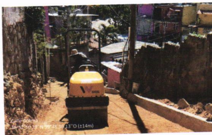
FORMACIÓN DE BASE DE 20CM DE ESPESOR
