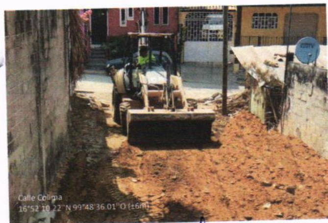
AFINE Y COMPACTACIÓN DE SUBRASANTE
