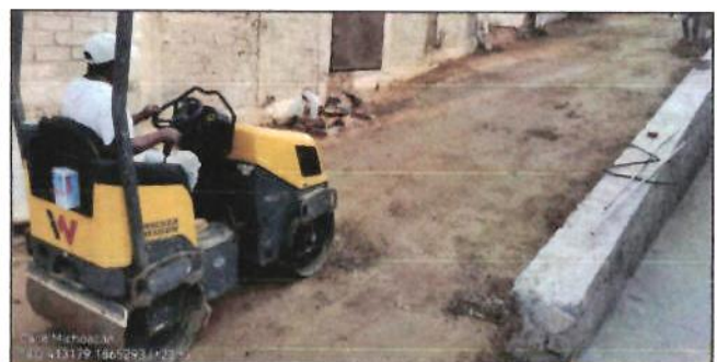
AFINE Y COMPACTACION DE SUBRASANTE AL 90 % PROCTOR
