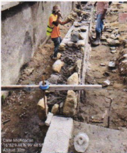
RODAPIE DE PIEDRA BRAZA DE LA REGION CON MEDIDAS DE 0.40 X 0.40 MTS
