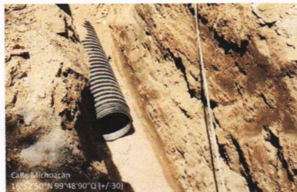
SUMINISTRO Y COLOCACION DE TUBERIA DE POLIETILENO DE 30 CMS DE DIAMETRO
