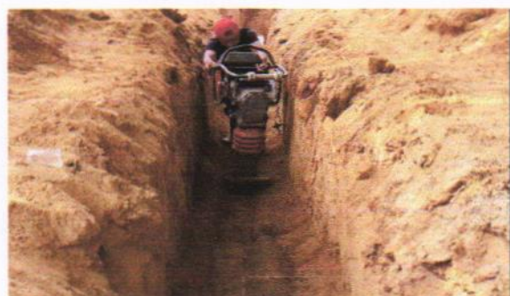
9-0138* RELLENO DE MATERIAL INERTE DE BANCO, COMPACTADO POR MEDIOS MECANICOS (BAILARINA) Y AGUA, EN CAPAS DE 20.00 cm. DE ESPESOR, INC.ACARREO DENTRO DE LA OBRA, MEDIDO COMPACTADO.
