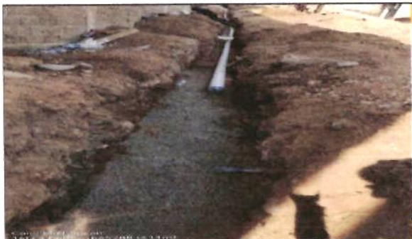
5-0102 CAMA DE ARENA PARA INSTALACION DE TUBERIA, INCLUYE: ACOSTILLADO, ACARREO DE MATERIAL EN 1ra. ESTACION, MATERIAL Y MANO DE OBRA.
