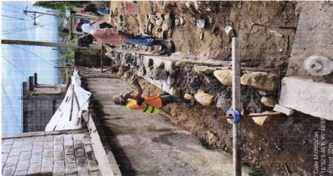
15-0283 RODAPIE DE PIEDRA BRAZA DE LA REGION CON MEDIDAS DE 0.40 X 0.40 MTS. ASENTADO CON MORTERO CEMENTO ARENA PROPORCIÓN 1:3 ACABADO COMUN INCLUYE: ACARREO, MATERIAL Y MANO DE OBRA.
