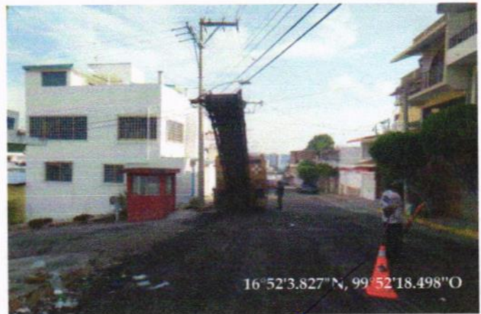
FRESADO DE CARPETA EXISTENTE
