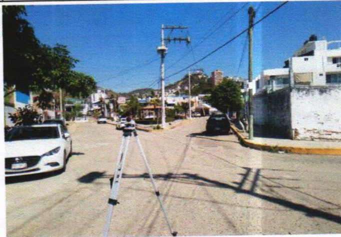
TRAZO Y NIVELACION TOPOGRAFICA DEL TERRENO
